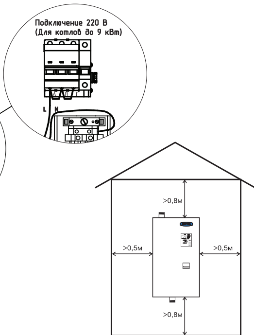
Рис. 4 Схема установки электроводонагревателя
