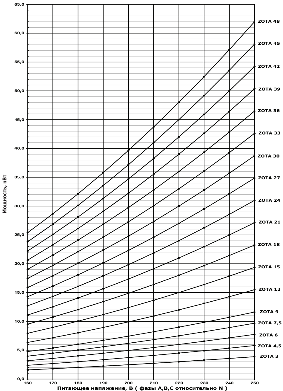
Рис. 11 График изменения мощности электроводонагревателя в зависимости от питающего напряжения стр.24
