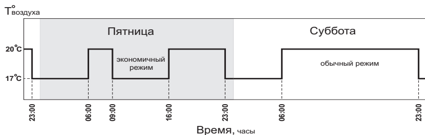
Рис. 7 График температуры воздуха в помещении для Режимы 3.
