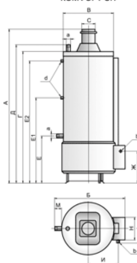
АОГВ-29-3; АКГВ-29-3 КОМФОРТ КОМФОРТ SIT
