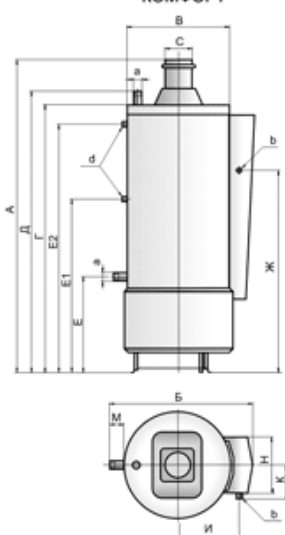
АОГВ-17,4-3; АКГВ-17,4-3 АОГВ-23,2-3; АКГВ-23,2-3 АОГВ-29-3; АКГВ-29-3 ЭКОНОМ, УНИВЕРСАЛ, КОМФОРТ
