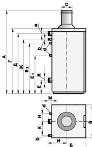
АОГВ-11,6-3 АКГВ-11,6-3 КОМФОРТ, Квадратный
