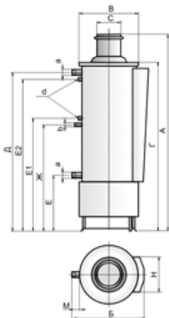
АОГВ-11,6-3 АКГВ-11,6-3 ЭКОНОМ
