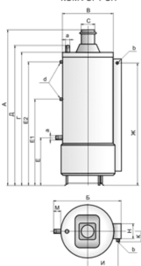
АОГВ-17,4-3; АКГВ-17,4-3 АОГВ-23,2-3; АКГВ-23,2-3 КОМФОРТ SIT
