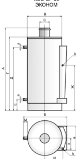
КОВ-СГ-43 КОВ-СГ-50 ЭКОНОМ
