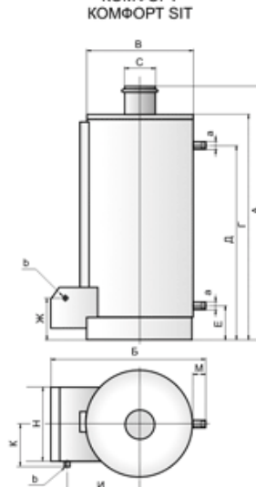
КОВ-СГ-43 КОВ-СГ-50 КОМФОРТ SIT
