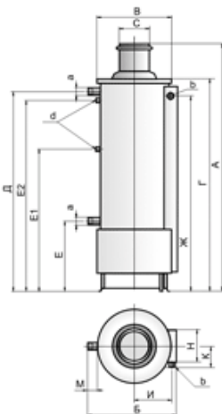
АОГВ-11,6-3 АКГВ-11,6-3 КОМФОРТ SIT
