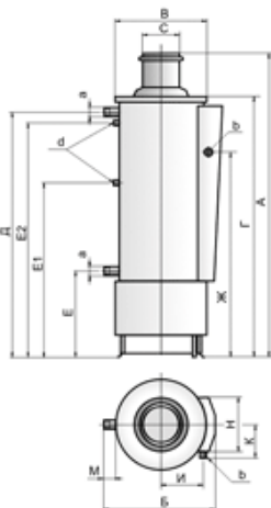
АОГВ-11,6-3 АКГВ-11,6-3 КОМФОРТ
