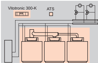
■ трехкотловая установка
